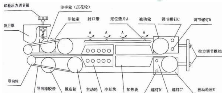
封口原理图
